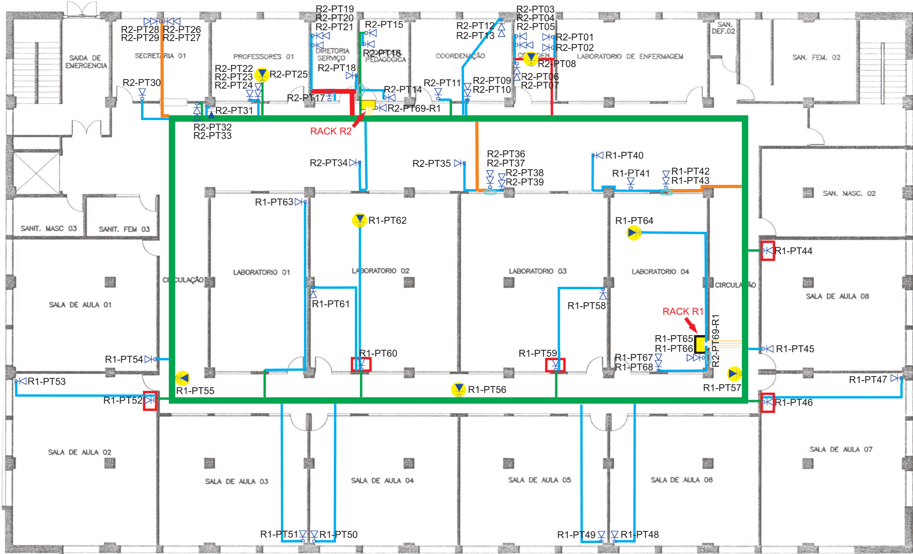
PLANTA 1º PAVIMENTO ( ETEC ANTONIO DEVISATE) ESC.1:100
