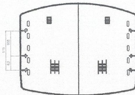
VISTA INFERIOR DO ASSENTO
