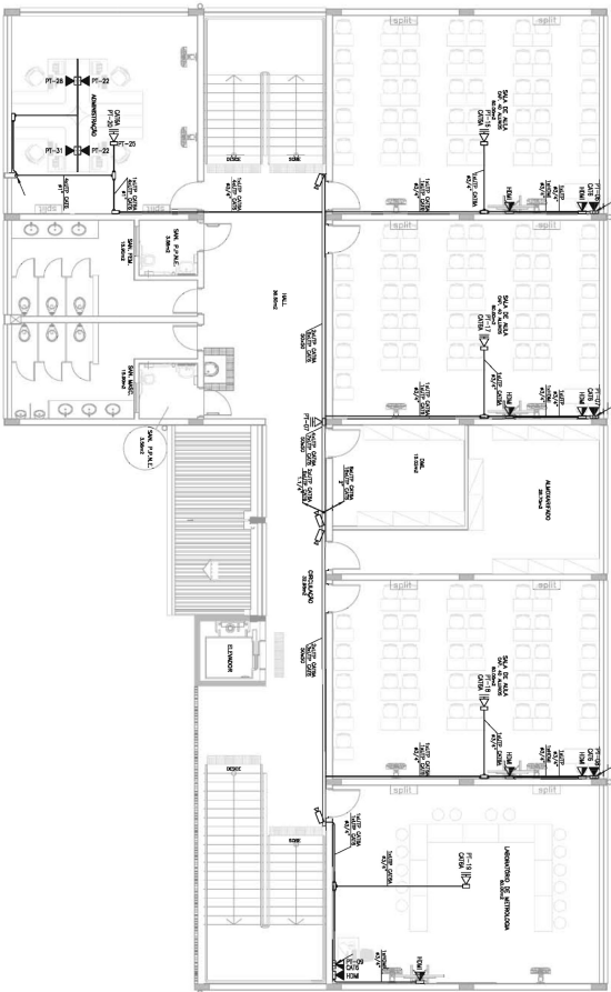
PLANTA 1º PAVIMENTO ESC. 1/100
