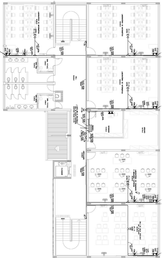
PLANTA 2º PAVIMENTO ESC. 1/100
