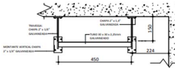
DETALHE ESC: 1 : 10
