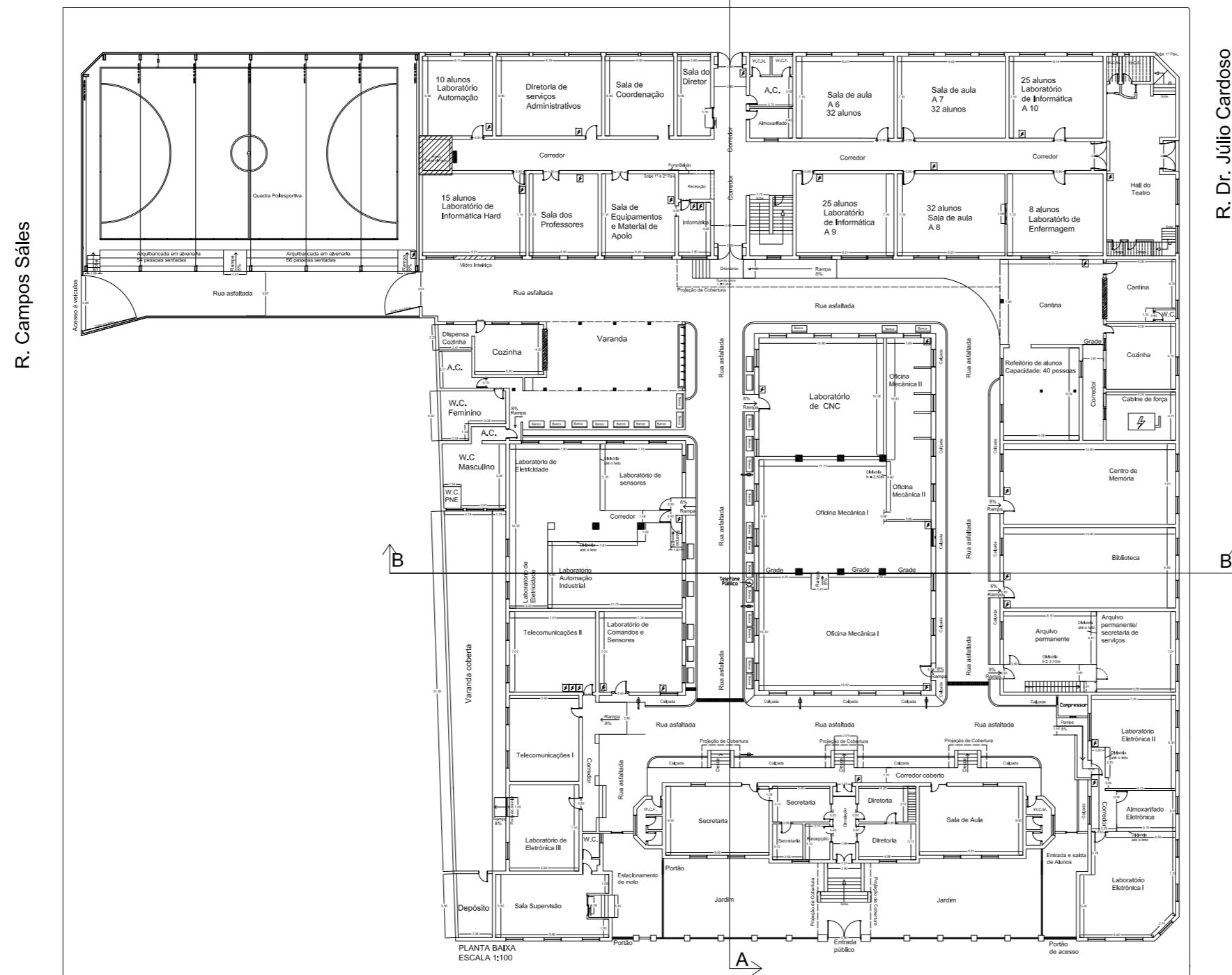
PLANTA BAIXA - PRIMEIRO PAVIMENTO ESCALA 1:100
