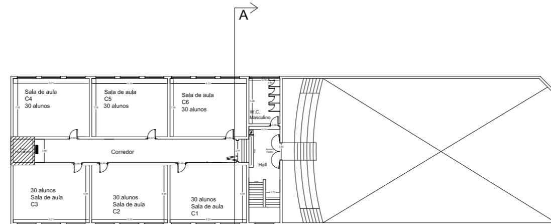
PLANTA BAIXA - SEGUNDO PAVIMENTO ESCALA 1:100
