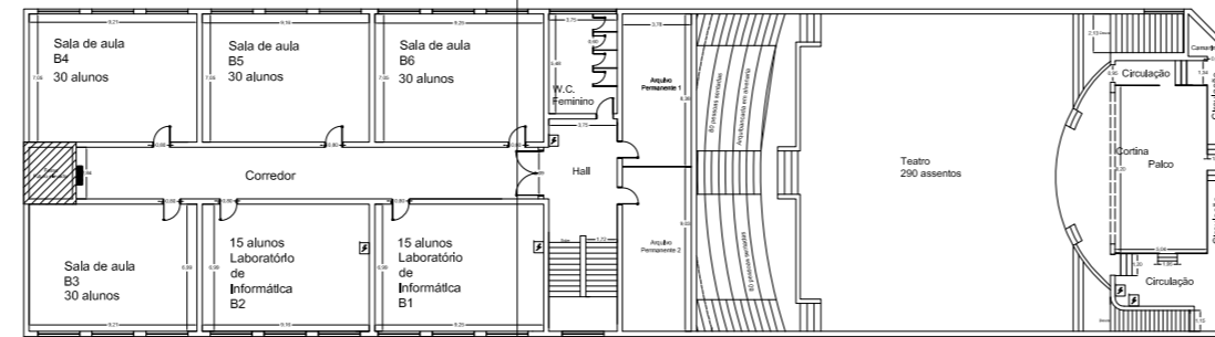
PLANTA BAIXA - PRIMEIRO PAVIMENTO ESCALA 1:100
