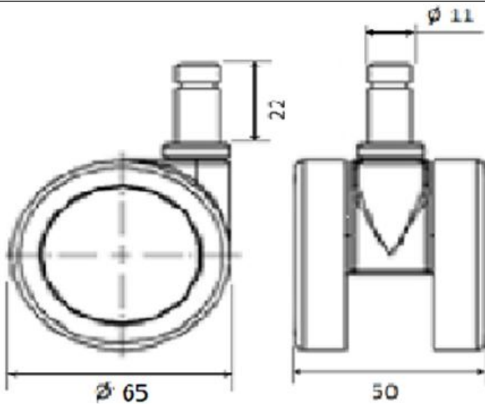
Imagem 01: Desenho técnico do rodízio
