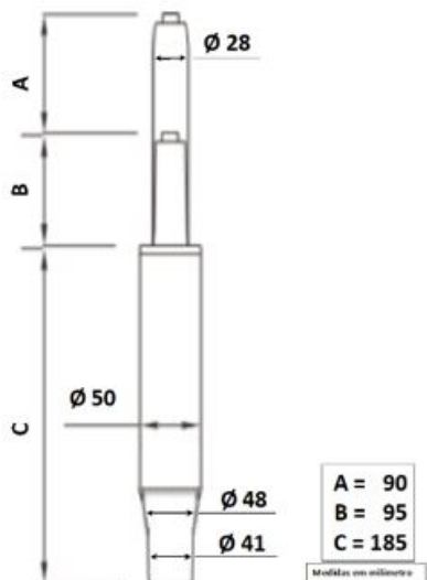
Imagem 05: Desenho técnico da coluna a gás
