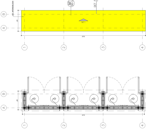
ABRIGO DE GÁS PLANTA CORREDOR IMPERMEABILIZAÇÃO DO TIPO 1 ESCALA 1/25
