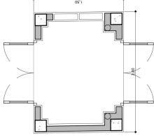
LUXEIRA PLANTA CORREDOR IMPERMEABILIZAÇÃO DO TIPO 1 ESCALA 1/25
