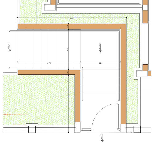
ESCALA DE ACESSO (LUNDOS) PLANTA CORREDOR IMPERMEABILIZAÇÃO DO TIPO 1 ESCALA 1/25
