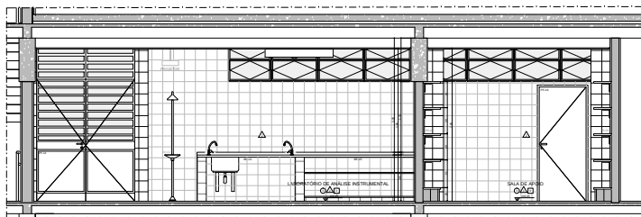
LABORATÓRIO DE ANÁLISE INSTRUMENTAL | ELEVACÃO 1
