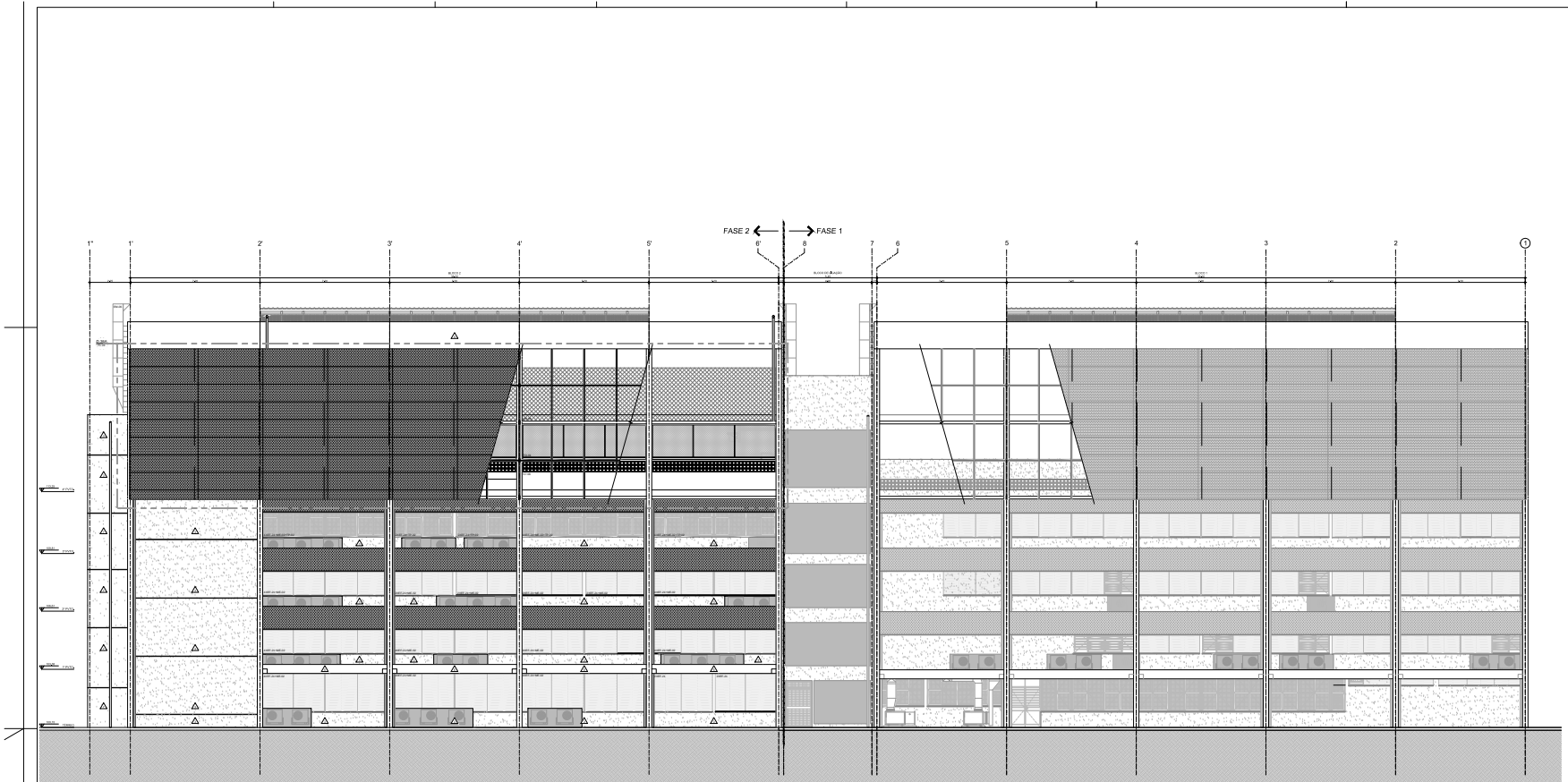
ELEVACÃO 2
