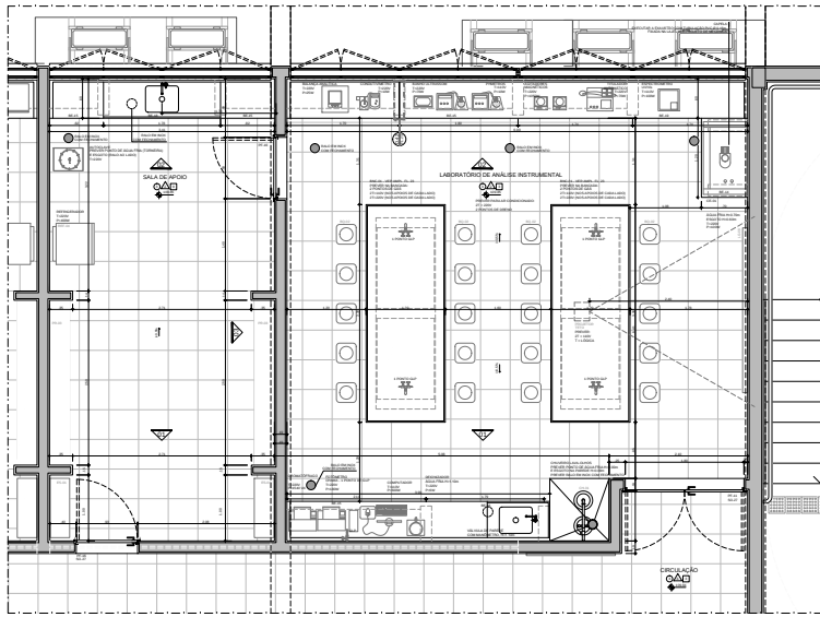
AMP-02 - LABORATÓRIO DE ANÁLISE INSTRUMENTAL | PLANTA
