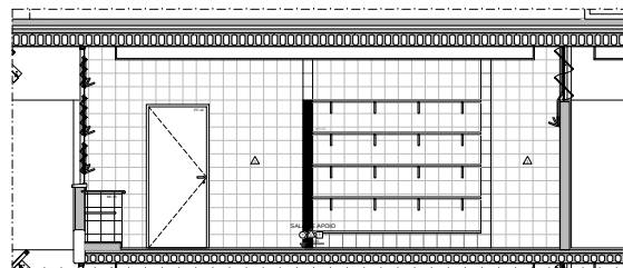
AMP-02 - LABORATÓRIO DE ANÁLISE INSTRUMENTAL | ELEVACÃO 3
