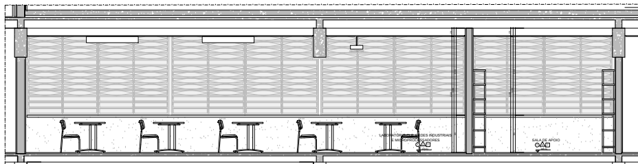
AMP-04 - LABORATÓRIO DE CLP, REDES INDUSTRIAIS E MICROPROCESSADORES | ELEVÇÃO 2
