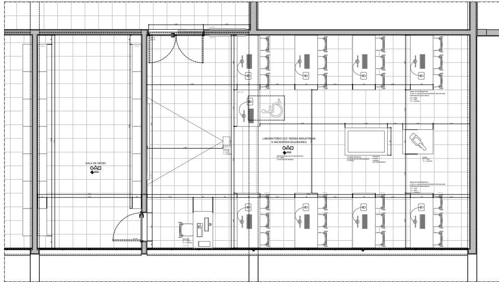
AMP-04 - LABORATÓRIO DE CLP, REDES INDUSTRIAIS E MICROPROCESSADORES - PLANTA
