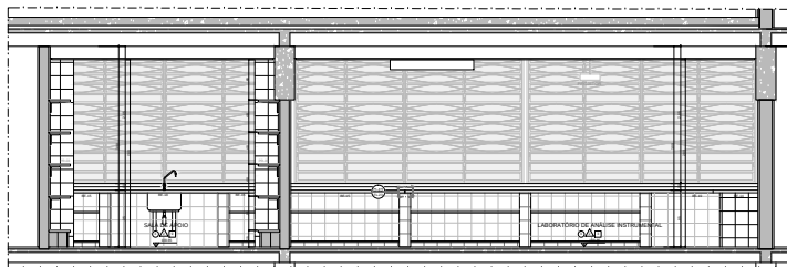
AMP-02 - LABORATÓRIO DE ANÁLISE INSTRUMENTAL | ELEVACÃO 2
