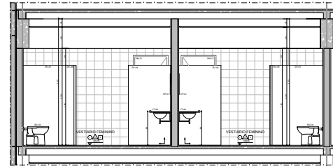
AMP 11 - VESTIÁRIOS 3º PVTO - CORTE AA
