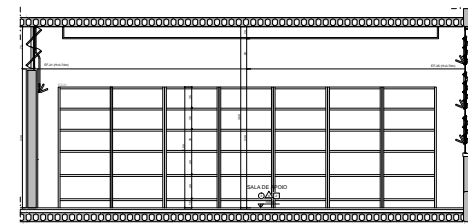
AMP-05 - LABORATÓRIO DE ELETRICIDADE E ELETRÔNICA - VISTA 02
