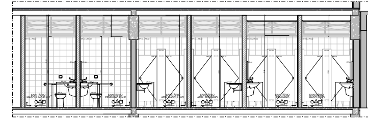
AMP 09 - CNUT. SANITÁRIOS 1º PVTO - CORTE AA
