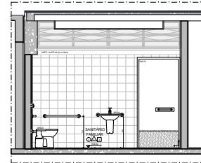
AMP 10 - CNUT. SANITÁRIOS 2º PVTO - CORTE BB
