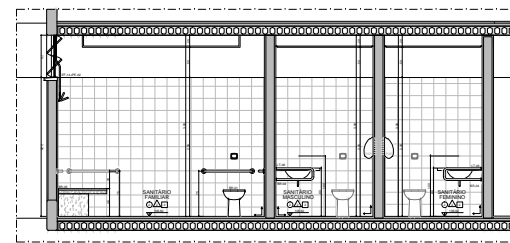
AMP 10 - CNUT. SANITÁRIOS 2º PVTO - CORTE AA
