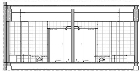
AMP 11 - VESTIÁRIOS 3º PVTO - CORTE BB
