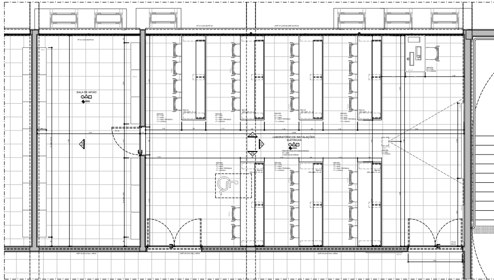
AMP-07 - LABORATÓRIO DE INSTALAÇÕES ELÉTRICAS - PLANTA
