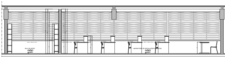
AMP-08 - LABORATÓRIO DE INSTALAÇÕES ELÉTRICAS - VISTA 01
