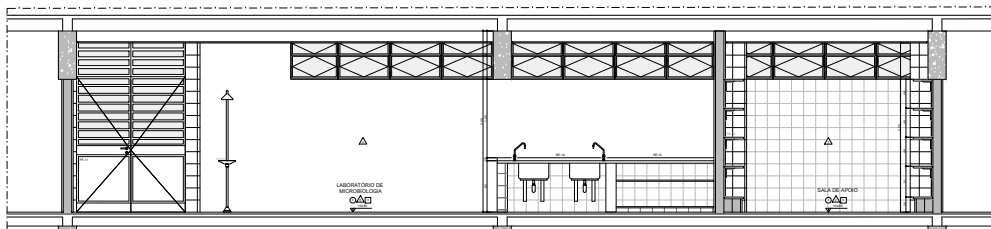
AMP-09 - LABORATÓRIO DE MICROBIOLOGIA | ELEVÇÃO 1
