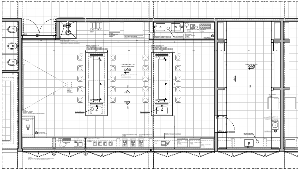
AMP-09 - LABORATÓRIO DE MICROBIOLOGIA | PLANTA
