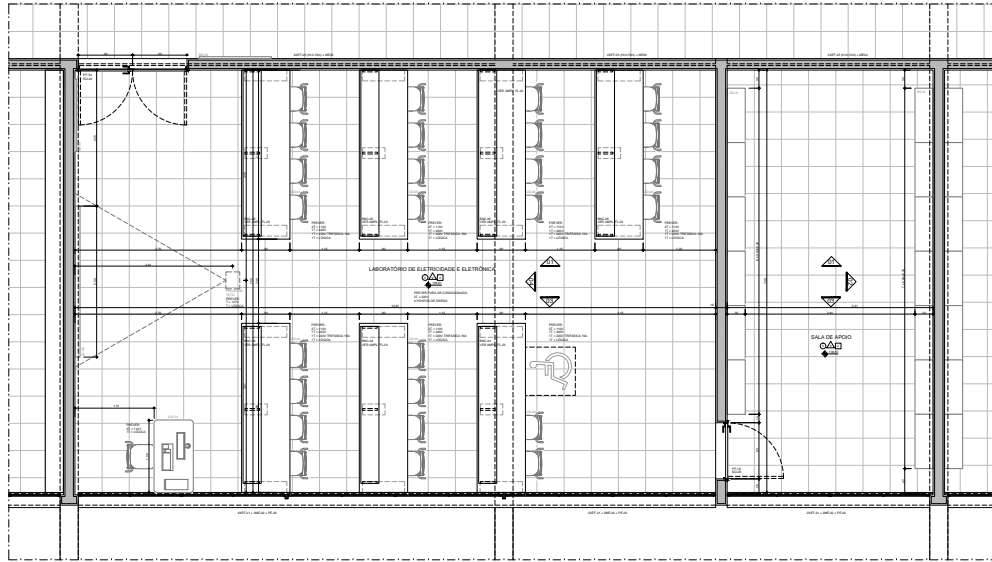
AMP-05 - LABORATÓRIO DE ELETRICIDADE E ELETRÔNICA - PLANTA
