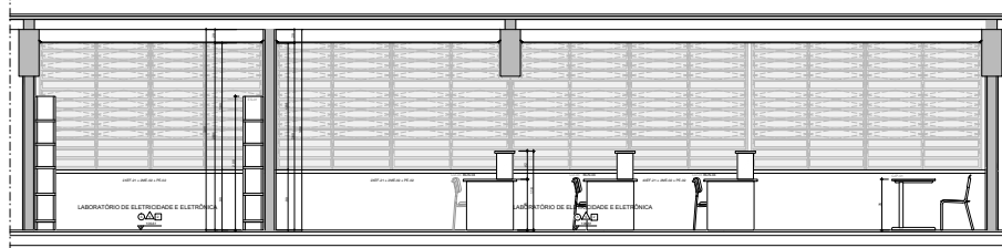
AMP-05 - LABORATÓRIO DE ELETRICIDADE E ELETRÔNICA - VISTA 03
