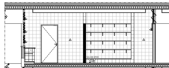
AMP-09 - LABORATÓRIO DE MICROBIOLOGIA | ELEVÇÃO 3
