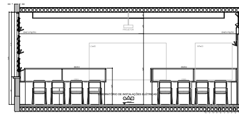
AMP-09 - LABORATÓRIO DE INSTALAÇÕES ELÉTRICAS - VISTA 02
