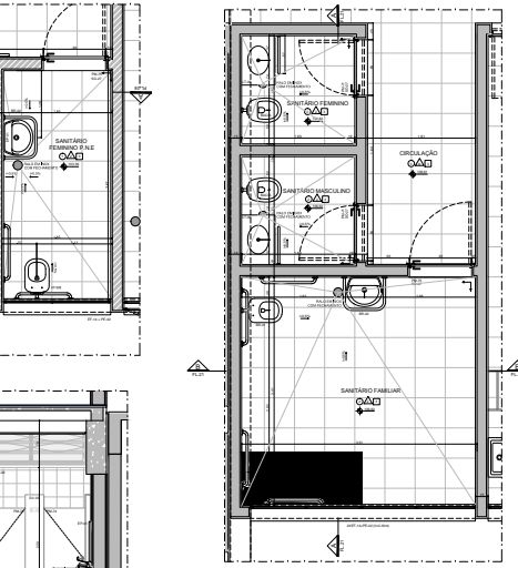
AMP 10 - CNUT. SANITÁRIOS 2º PVTO
