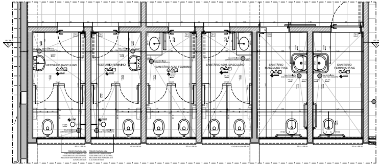
AMP 09 - CNUT. SANITÁRIOS 1º PVTO
