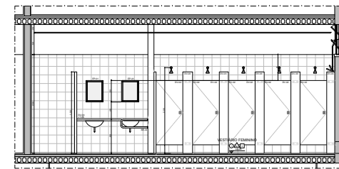
AMP 11 - VESTIÁRIOS 3º PVTO - CORTE CC
