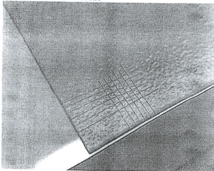
Figura 2 – Resultado 5B do ensaio ASTM D3359
