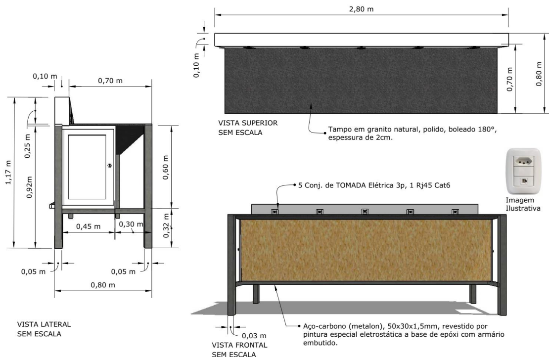
Figura – 1: Vista frontal, lateral e superior da bancada.
