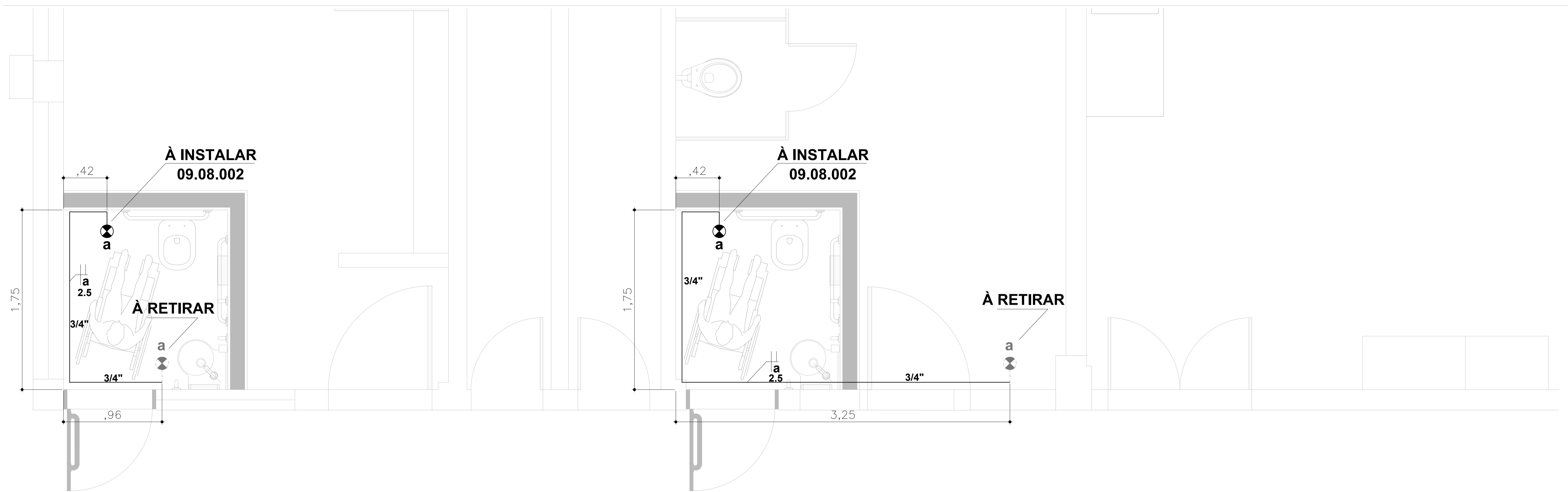
AMPLIAÇÃO 001A- SANITÁRIO ACESSÍVEL 1A PAVIMENTO TÉRREO 1:20
