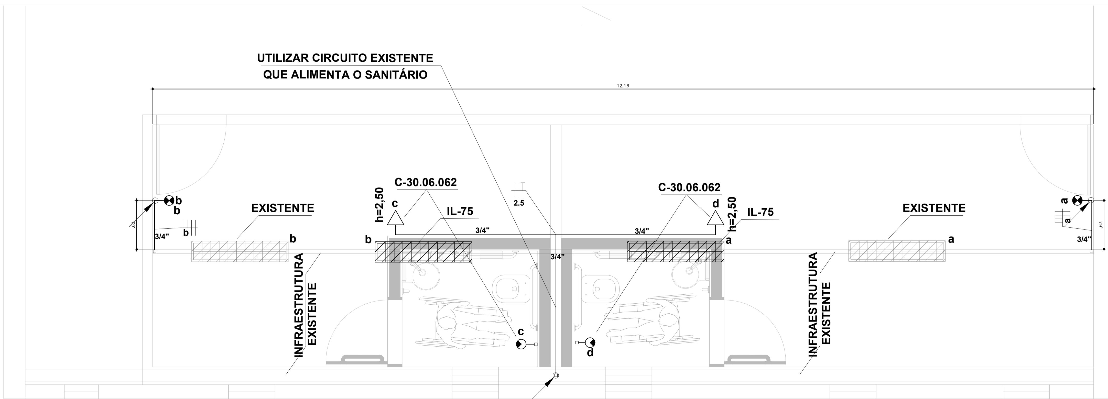
AMPLIAÇÃO 001A- SANITÁRIO ACESSÍVEL 1A PAVIMENTO TÉRREO 1:20
