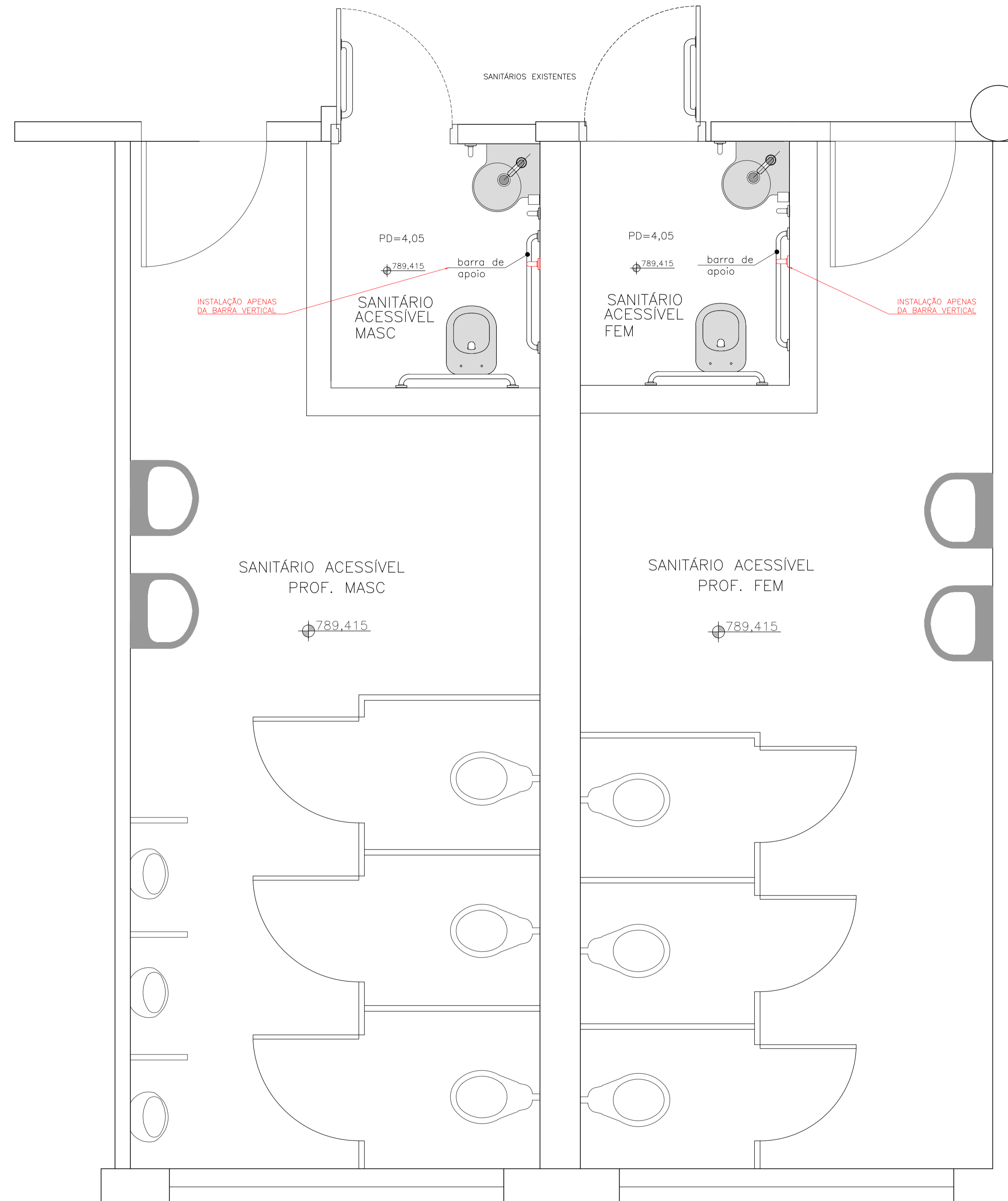
BLOCO A - SANITÁRIO - PLANTA EXISTENTE PAVIMENTO SUPERIOR 1:20
