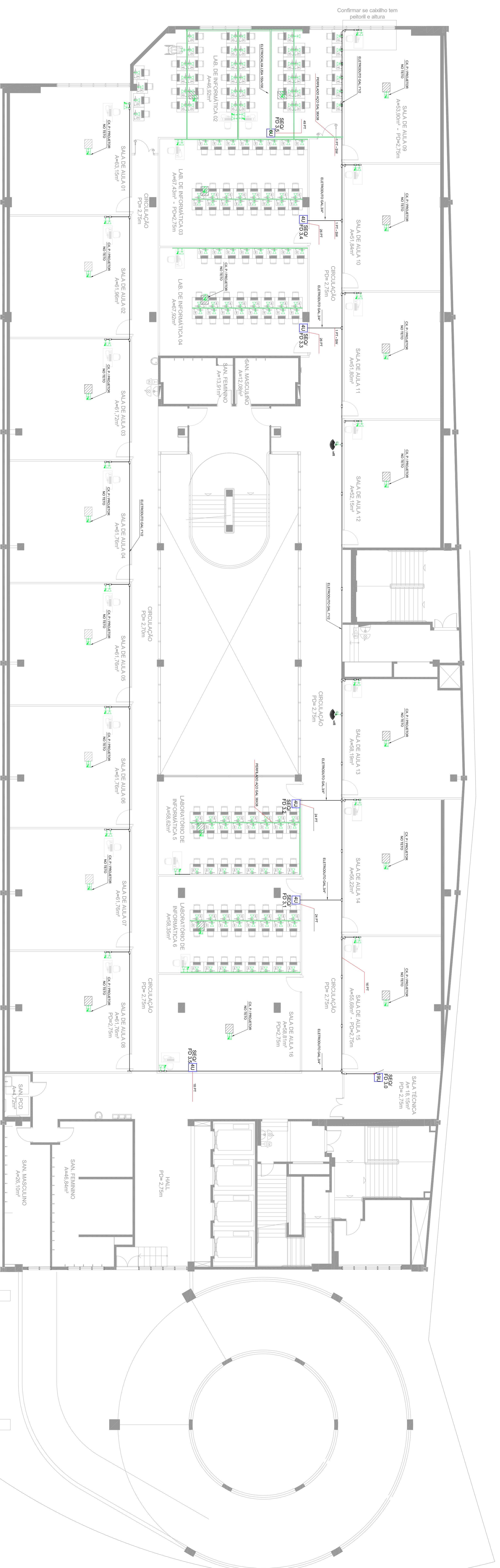
PLANTA DO 5º PAV. - FATEC ESCALA 1:100
