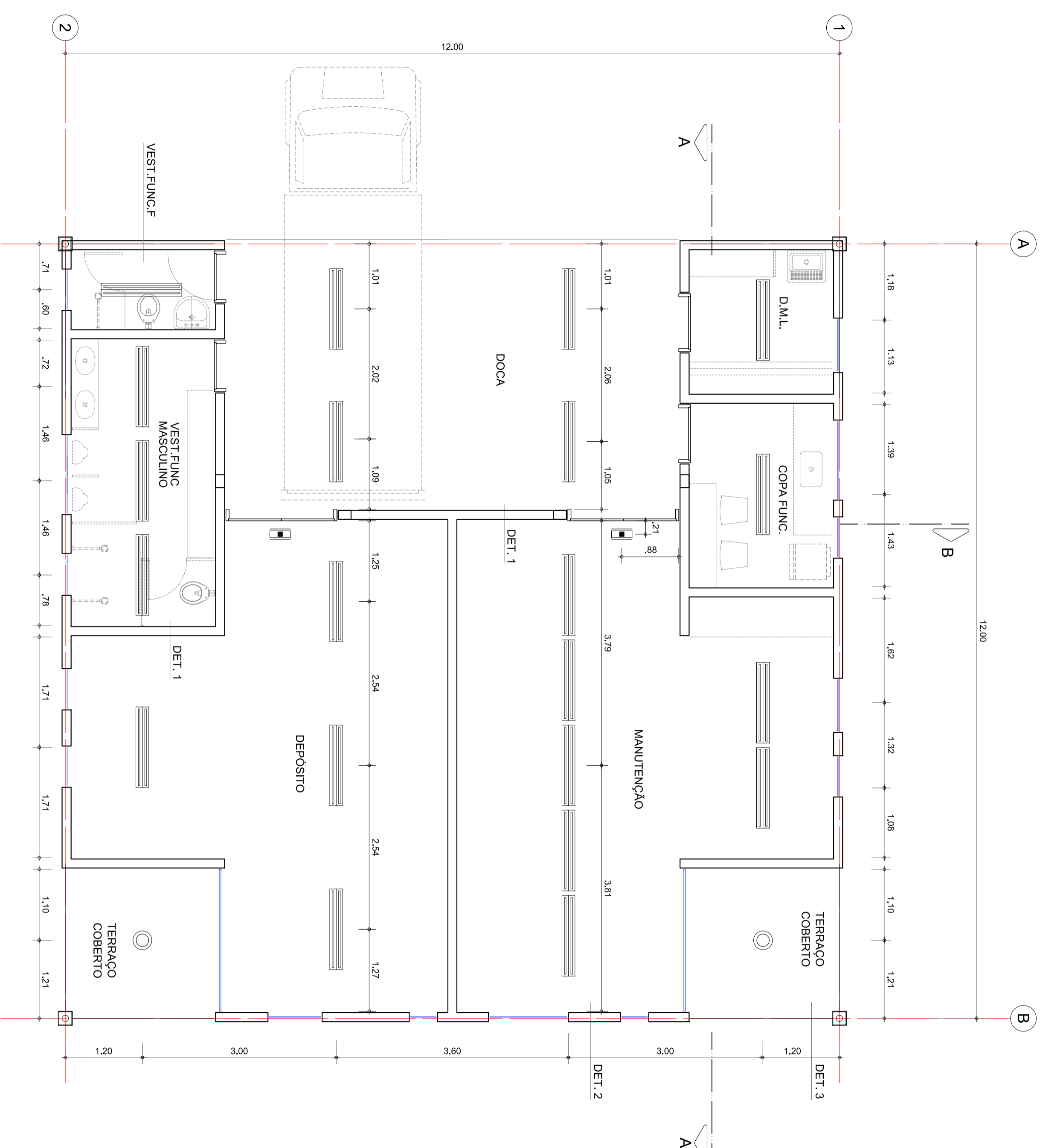
PLANTA DE FORRO ESCALA 1:50
