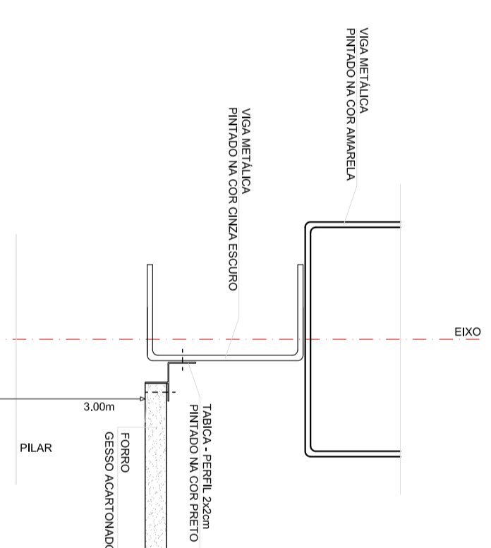
CORTE - DETALHE 3 (FORRO EXTERNO X VIGA)
