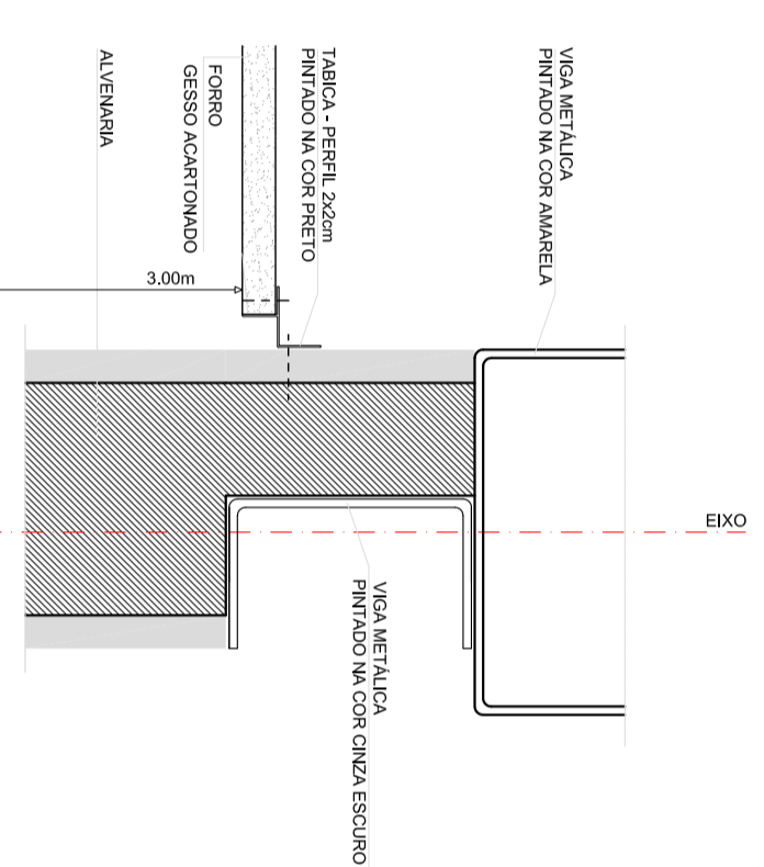
CORTE - DETALHE 2 (PARDE ALVENARIA EXTERNA x FORRO)
