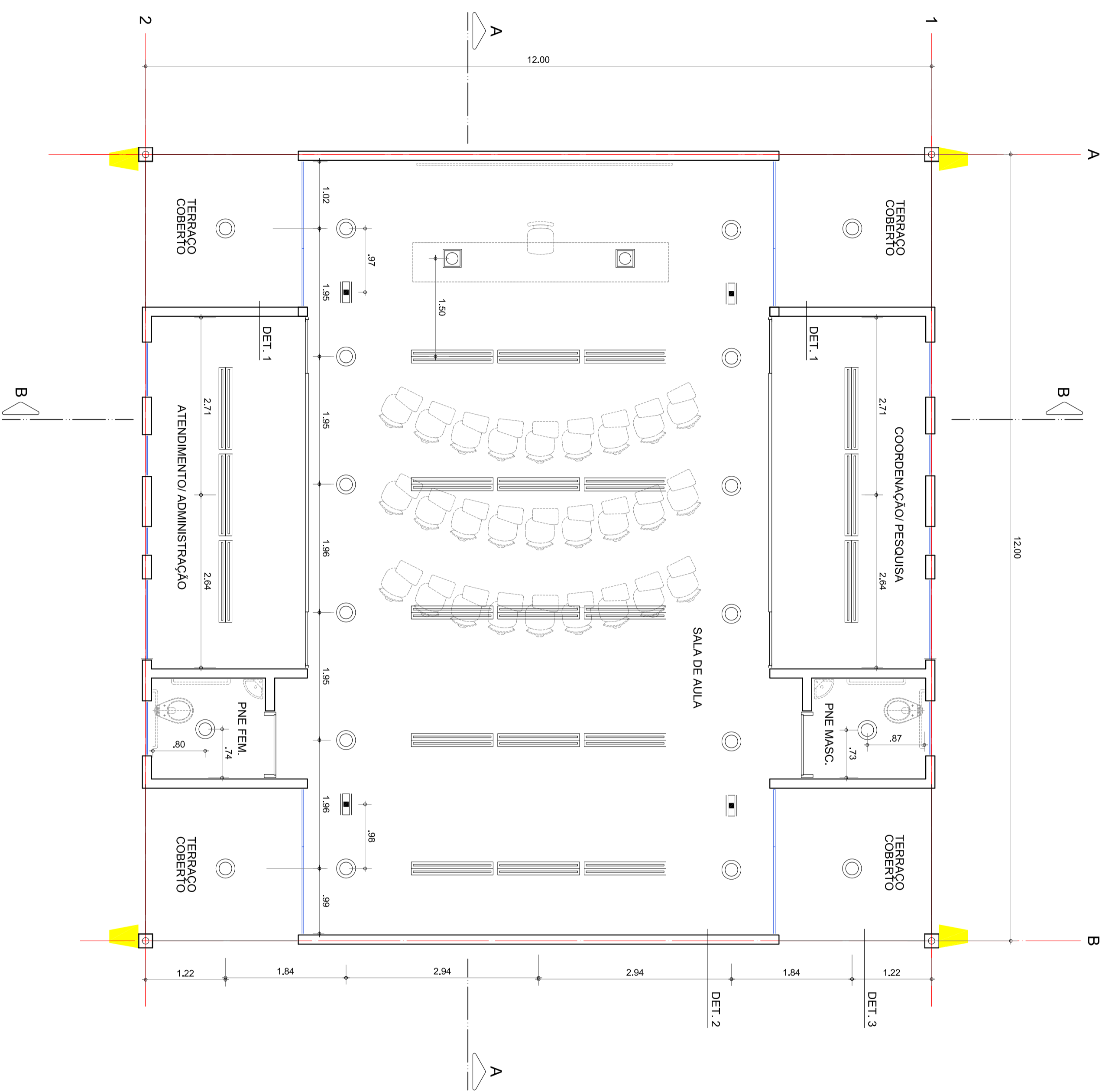
PLANTA DE FORRO ESCALA 1:50
