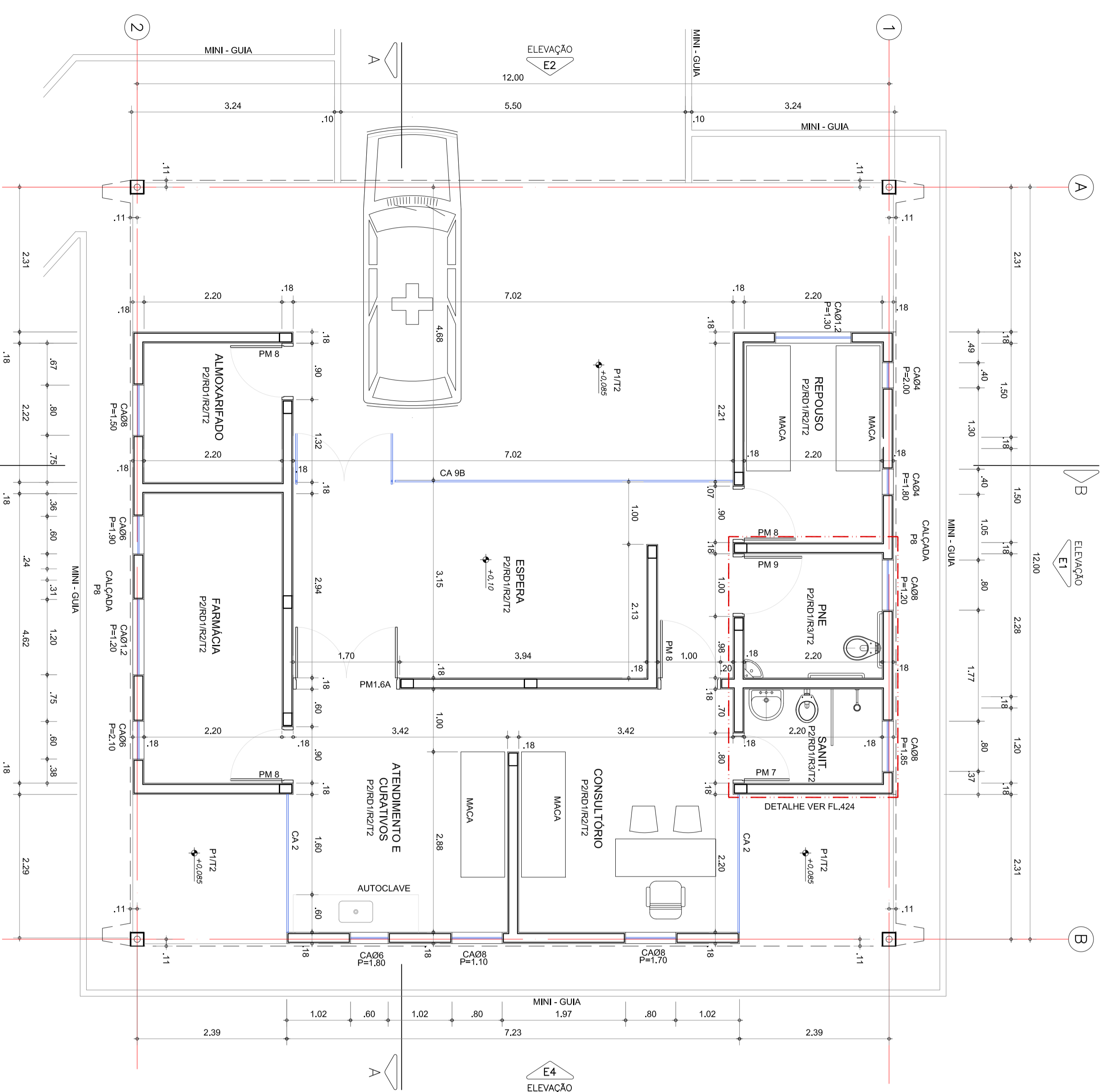
PLANTA ESCALA 1:50
