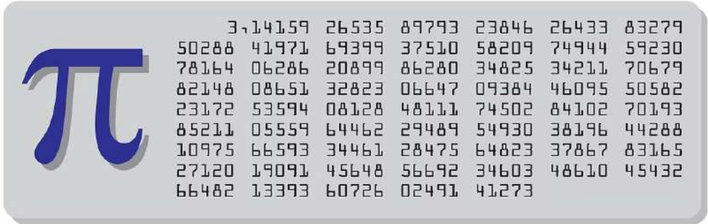
Número Pi com 300 casas decimais
