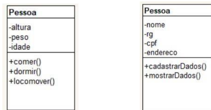
Figura 1 – Diagramas de classes utilizadas no exemplo Fonte: do autor
